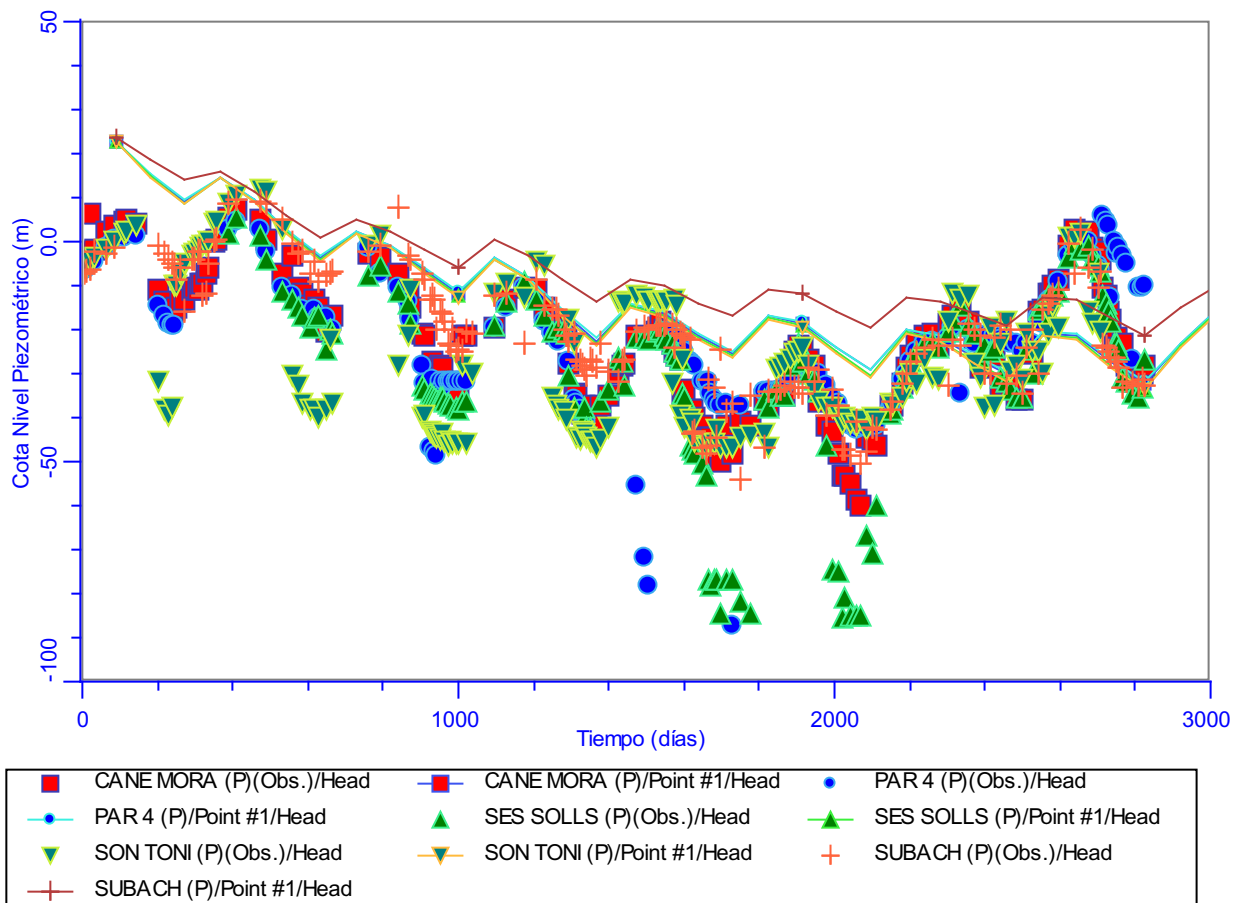
FIGURA 7B. CALIBRACIÓN DEL MODELO PARA POROSIDAD EFICAZ DEL 3%
