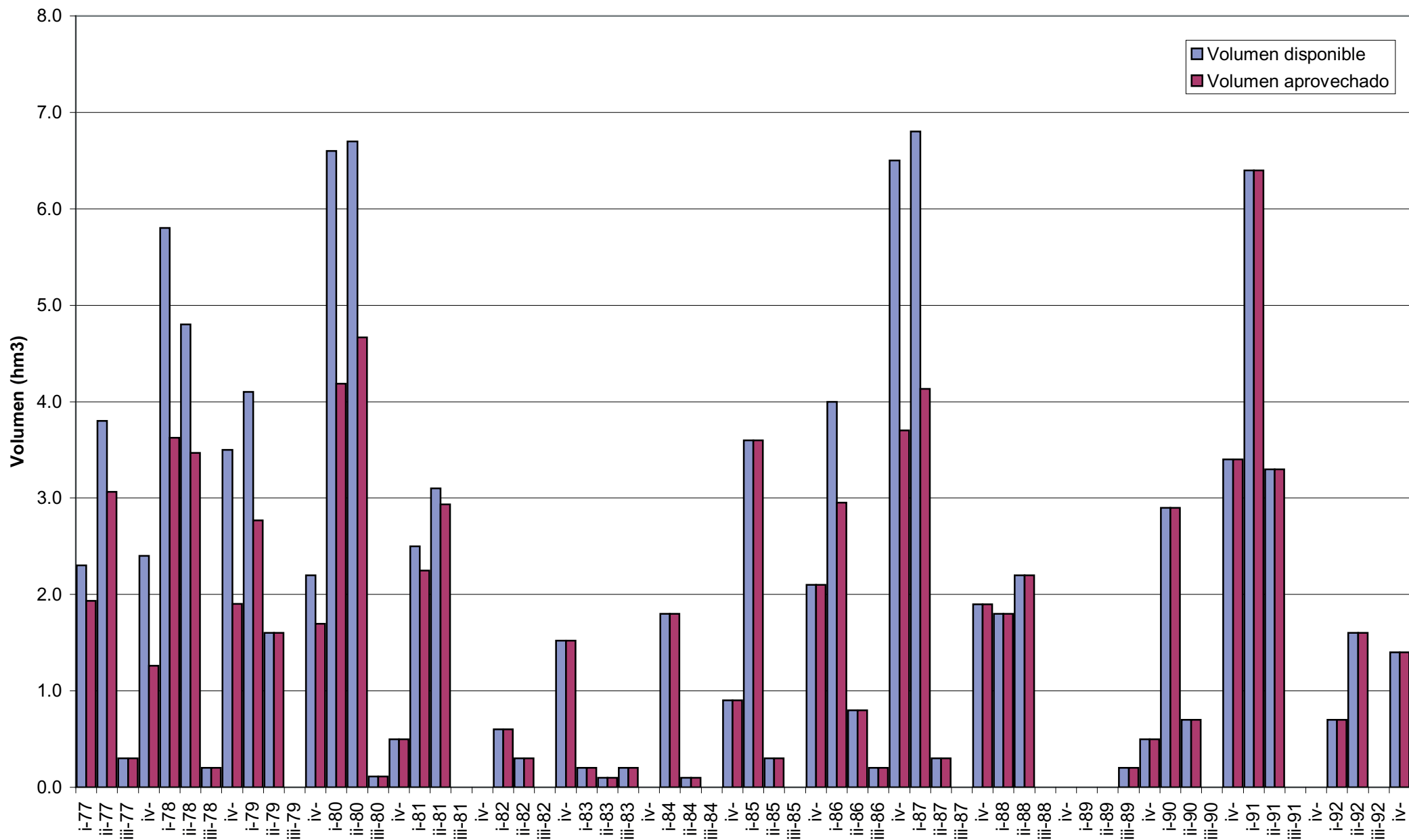
FIGURA 12. RELACIÓN TRIMESTRAL ENTRE VOLUMEN DISPONIBLE Y VOLUMEN APROVECHADO PARA RECARGA ARTIFICIAL
