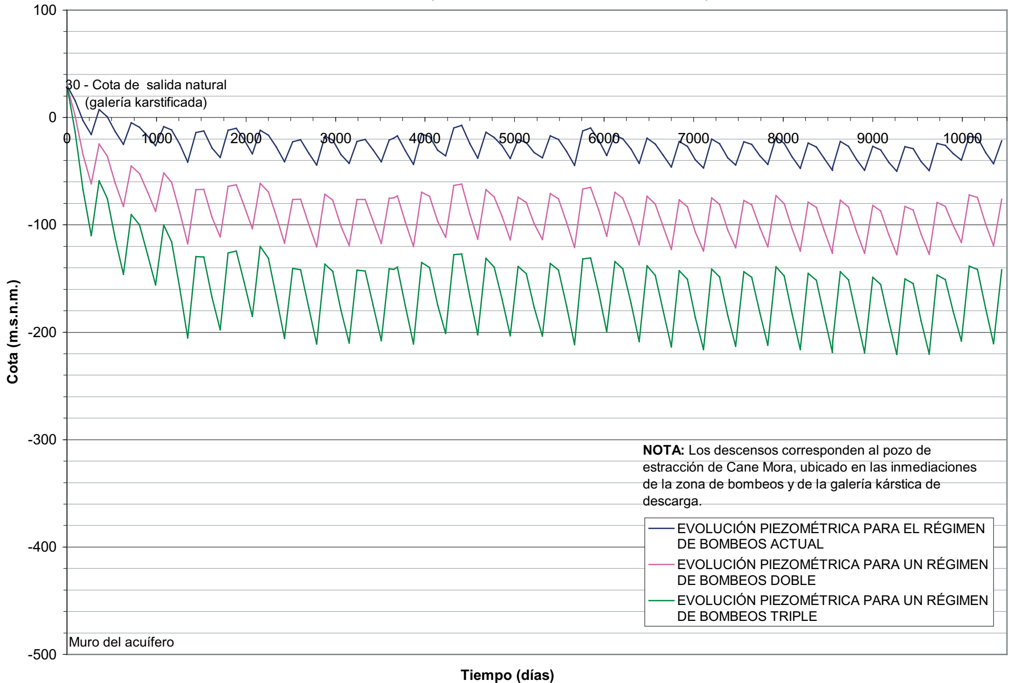
FIGURA 8. EVOLUCIÓN TEMPORAL ESTIMADA DE LOS NIVELES PIEZOMÉTRICOS EN EL ACUÍFERO DE CRESTATX (SEGÚN EL RÉGIMEN DE BOMBEO)
