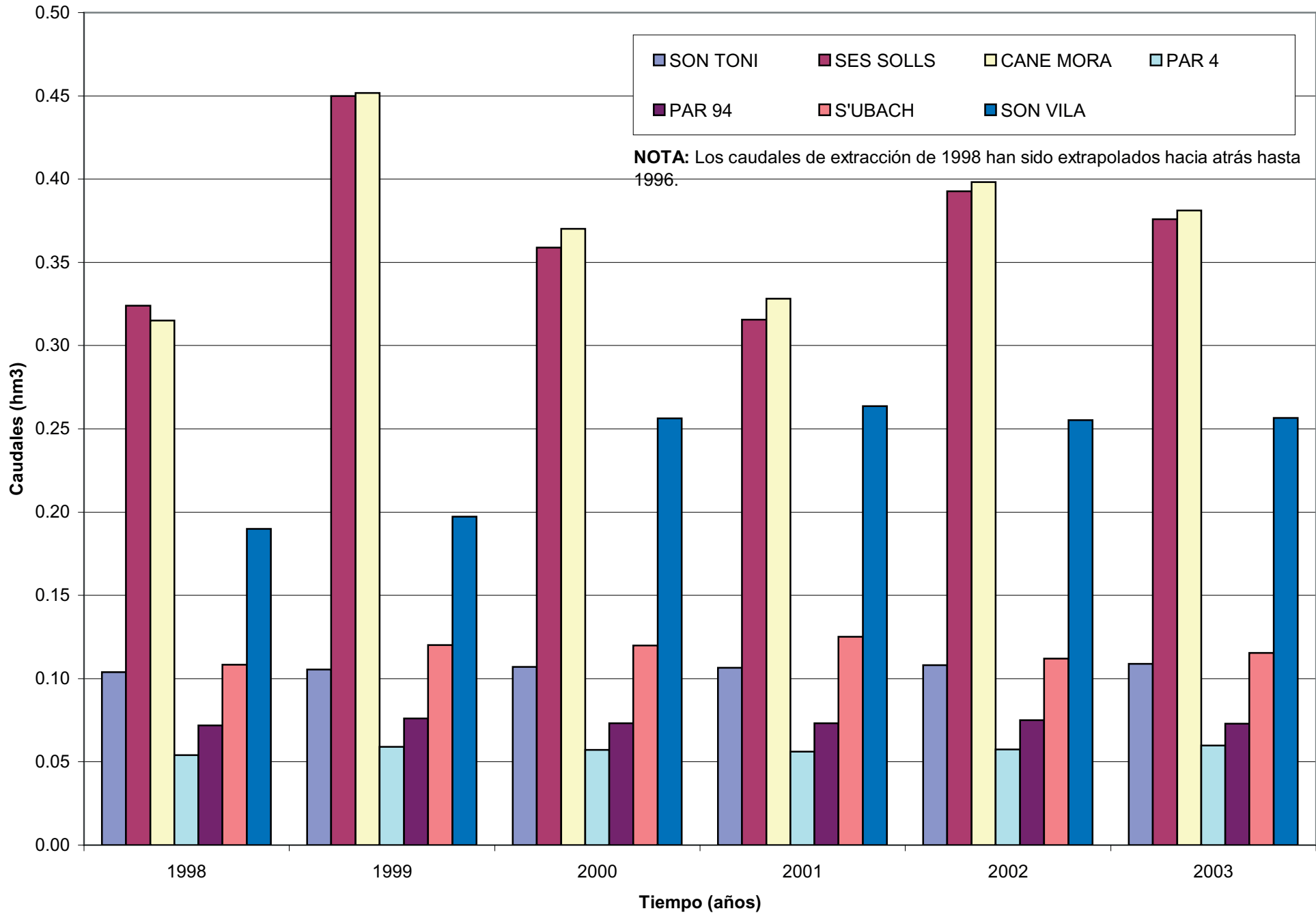
FIGURA 3. CAUDALES DE EXTRACCIÓN ANUALES POR POZOS
