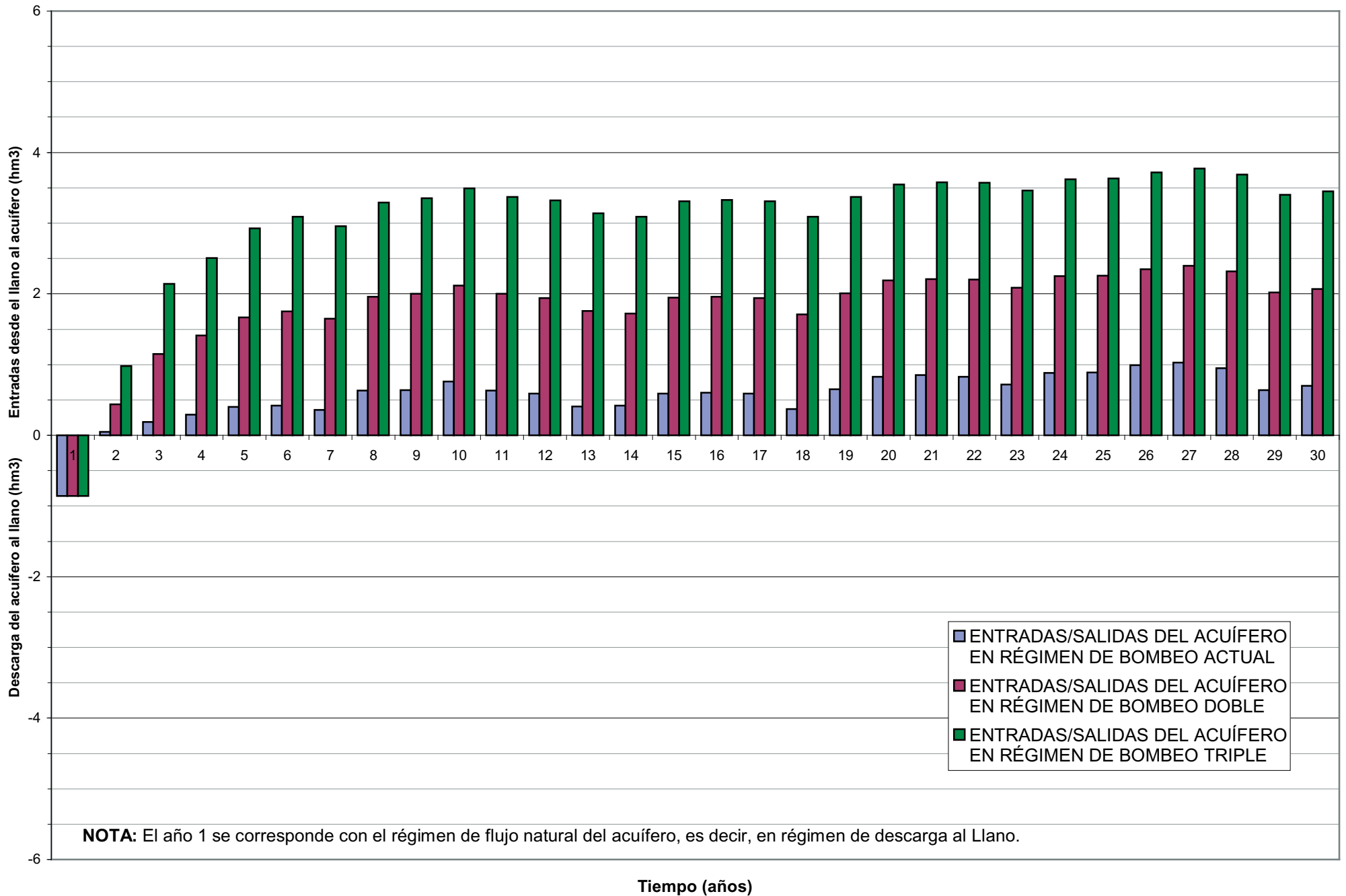
FIGURA 10. RELACIÓN ENTRE EL ACUÍFERO DE CRESTATX Y EL LLANO DE LA PUEBLA (SEGÚN EL RÉGIMEN DE BOMBEO)
