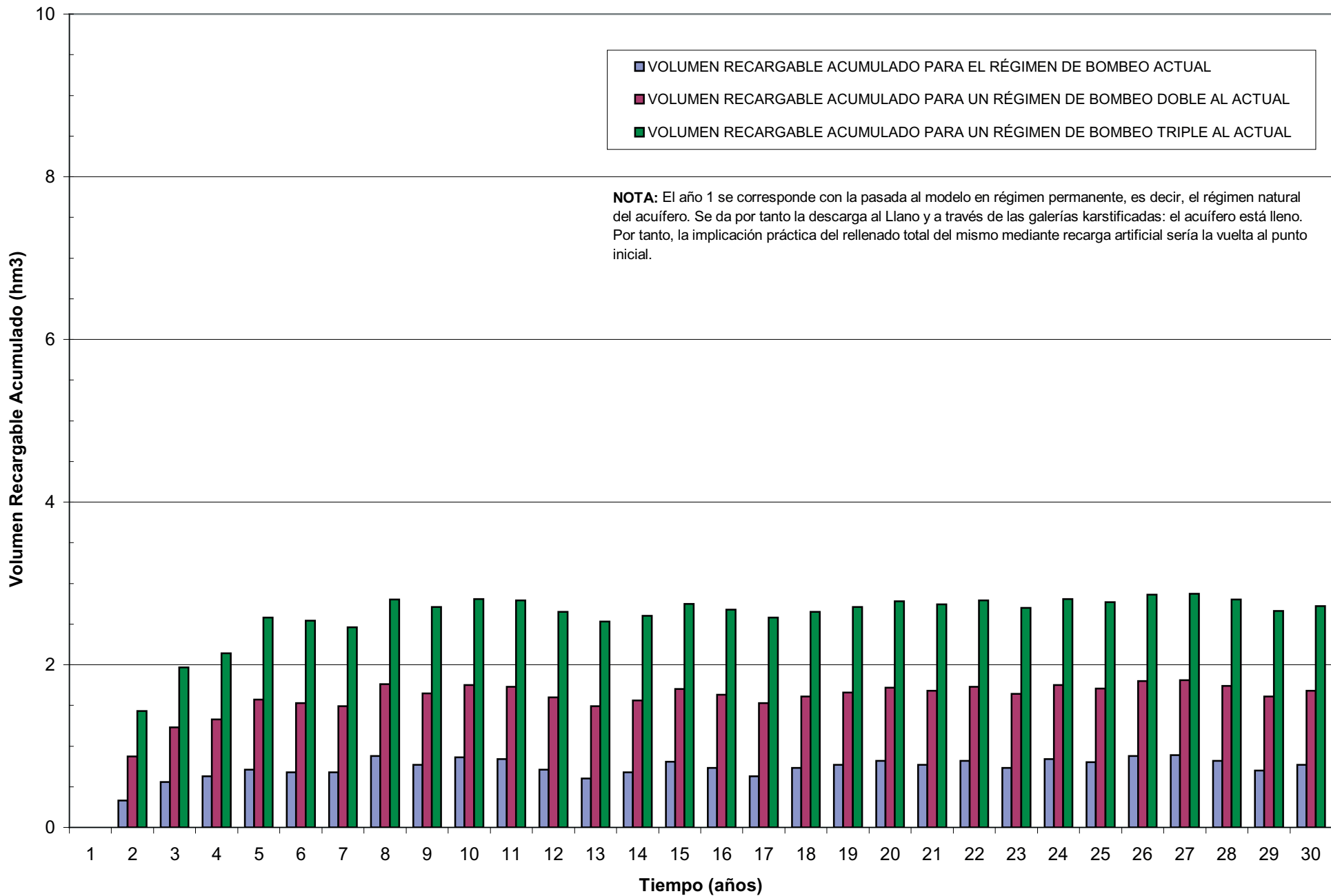
FIGURA 11. ESTIMACIÓN DEL VOLUMEN RECARGABLE EN EL TIEMPO PARA EL ACUÍFERO DE CRESTATX (SEGÚN EL RÉGIMEN DE BOMBEO)
