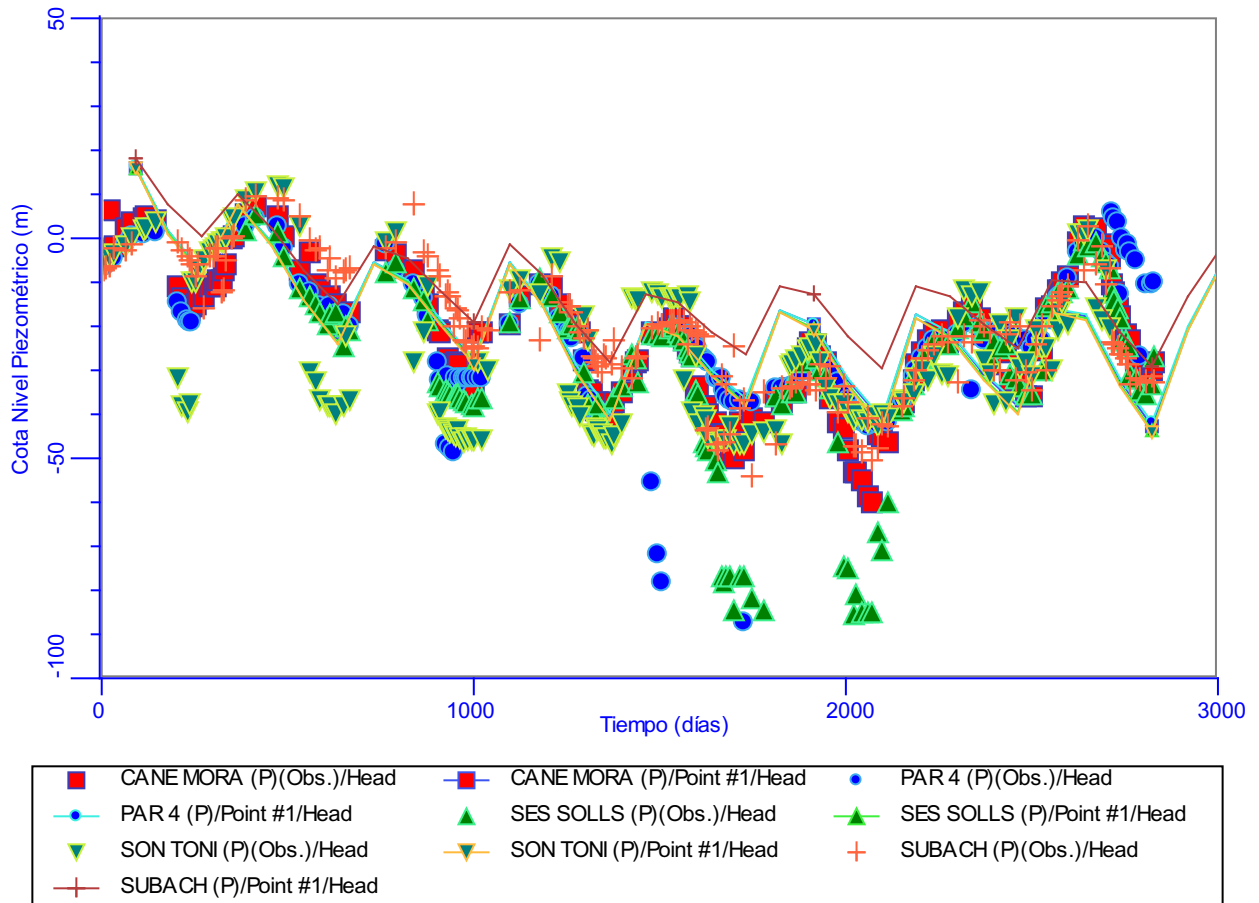
FIGURA 7A. CALIBRACIÓN DEL MODELO PARA POROSIDAD EFICAZ DEL 1%
