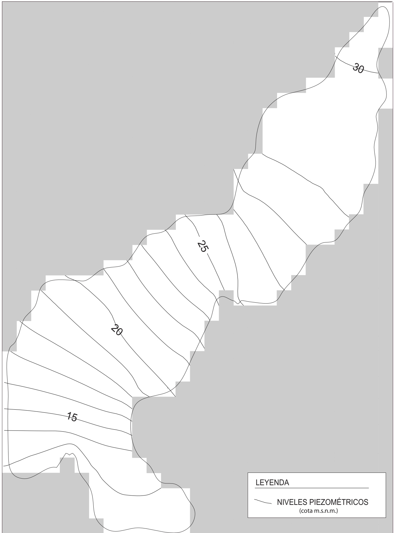
FIGURA 6. ISOPIEZAS EN RÉGIMEN NATURAL (PERMANENTE)
