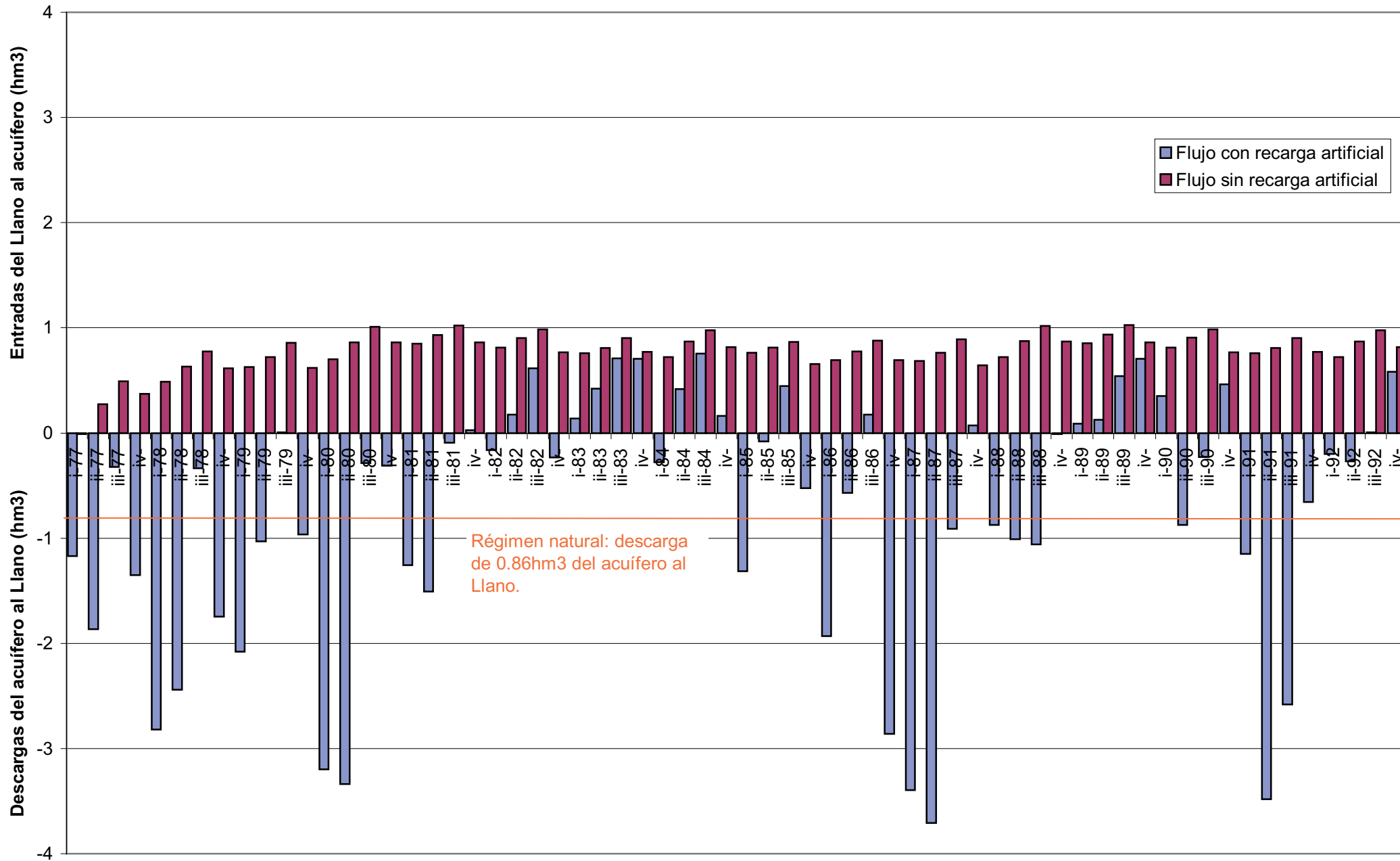
FIGURA 13. RELACIÓN DE TRIMESTRAL DE FLUJO ENTRE ACUÍFERO Y LLANO CON Y SIN RECARGA ARTIFICIAL
