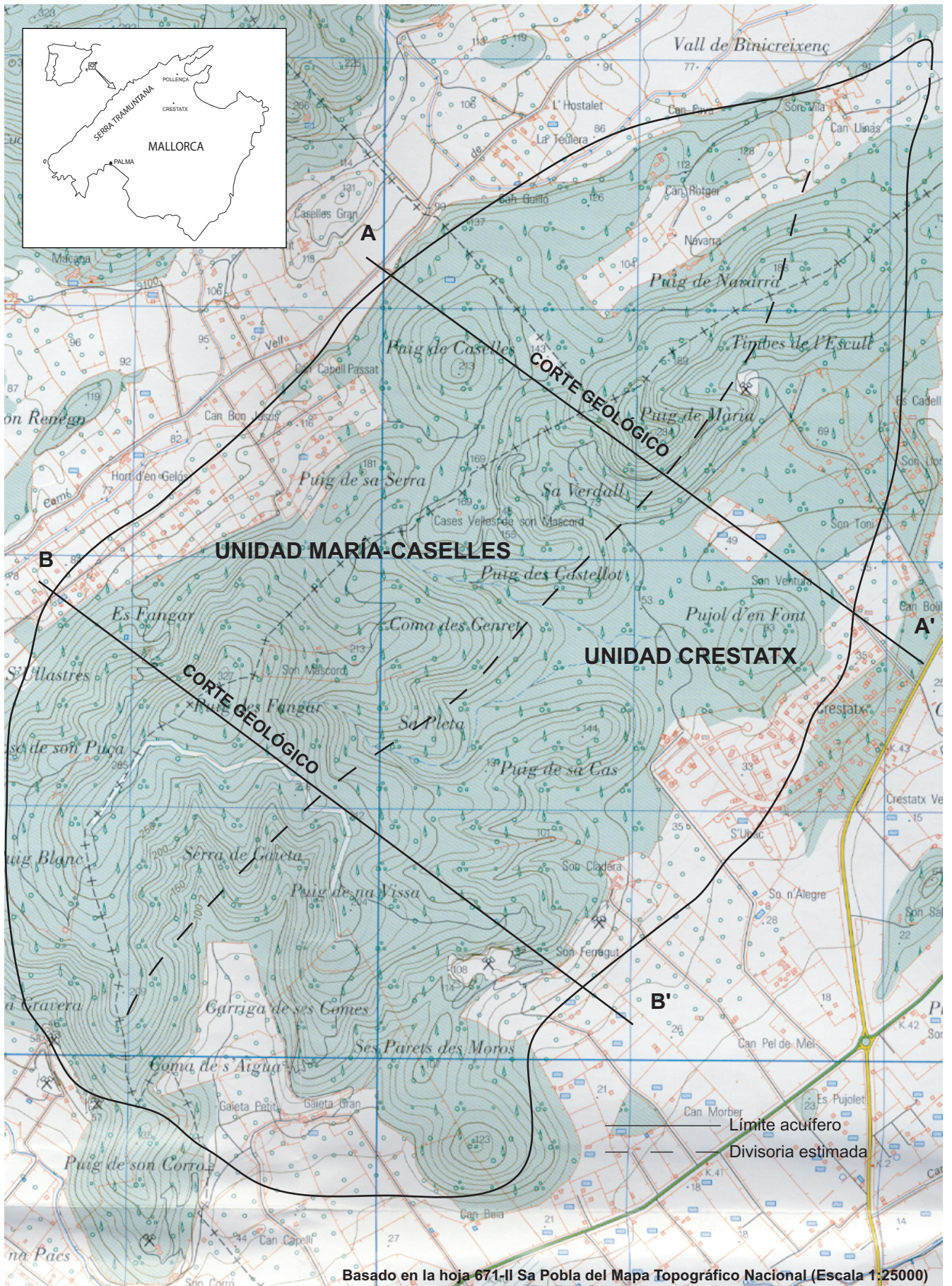
FIGURA 1. MAPA TOPOGRÁFICO Y DE SITUACIÓN DEL ACUÍFERO DE CRESTATX
