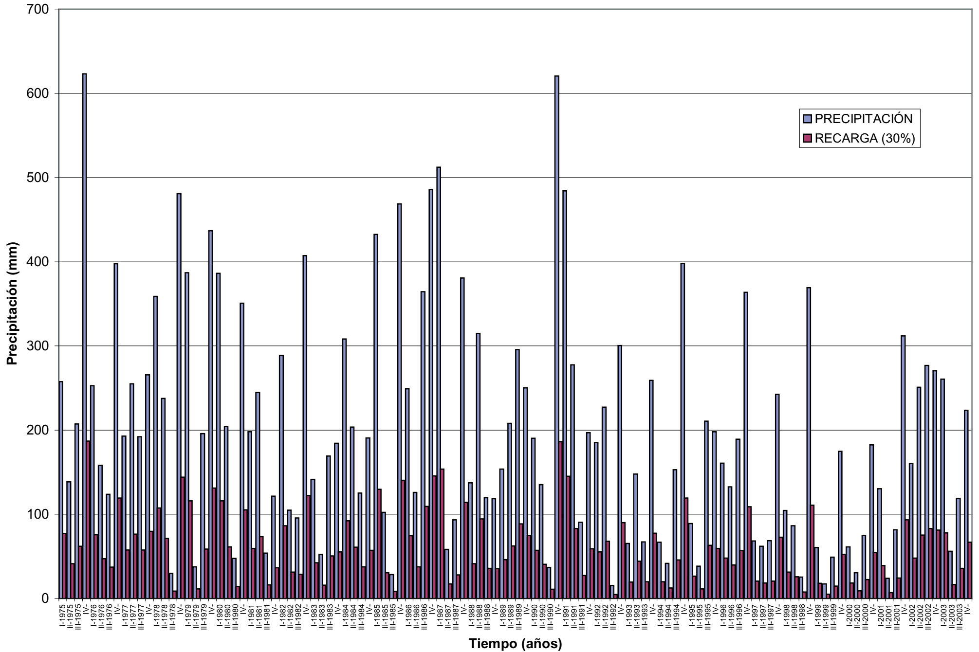
FIGURA 2. PRECIPITACIÓN TRIMESTRAL Y RECARGA ESTIMADA EN EL ACUÍFERO DE CRESTATX (1975-2003)
