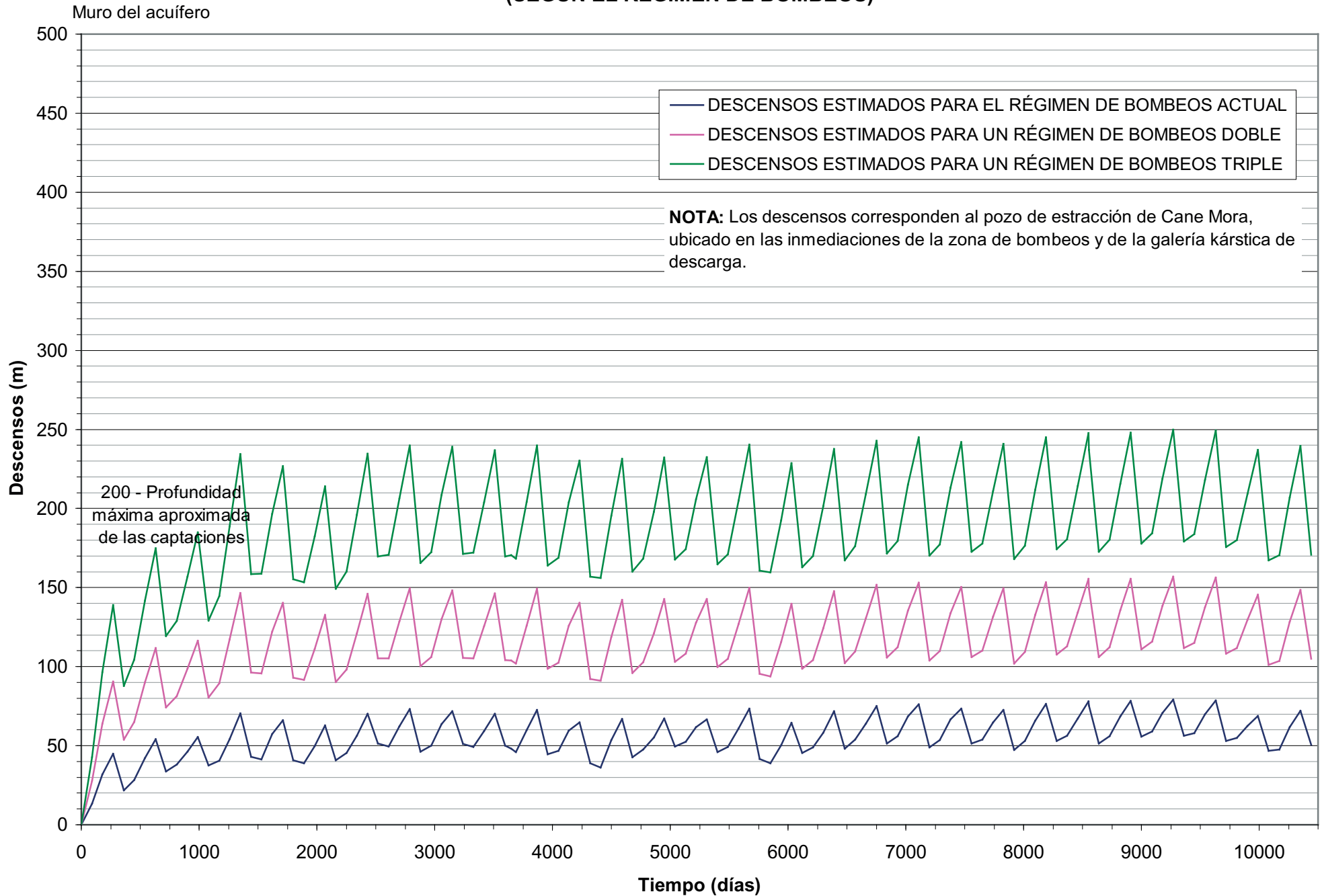
FIGURA 9. ESTIMACIÓN TEMPORAL DE LOS DESCENSOS EN EL ACUÍFERO DE CRESTATX (SEGÚN EL RÉGIMEN DE BOMBEO)
