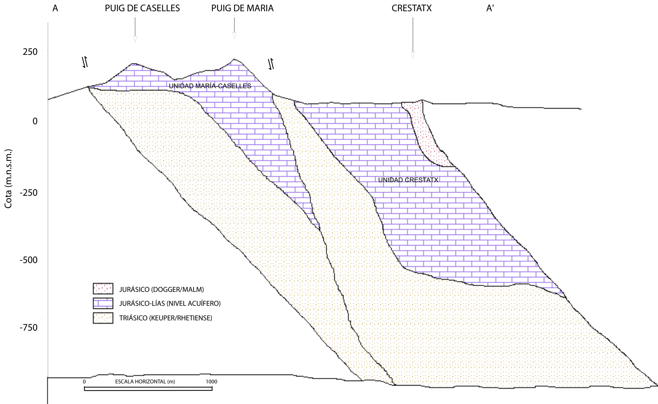
FIGURA 4. CORTE GEOLÓGICO A-A' DEL ACUÍFERO DE CRESTATX (Basado en Gelabert, 1997)
